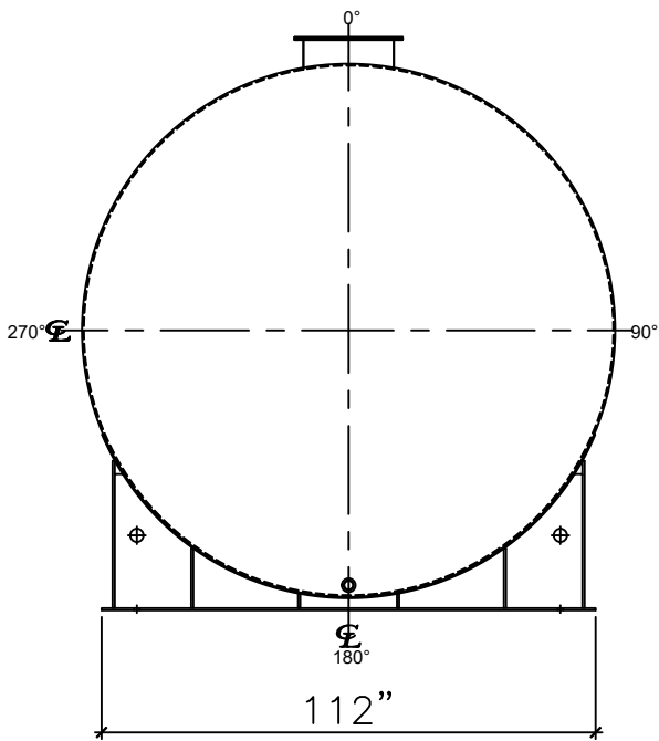
LEFT SIDE
