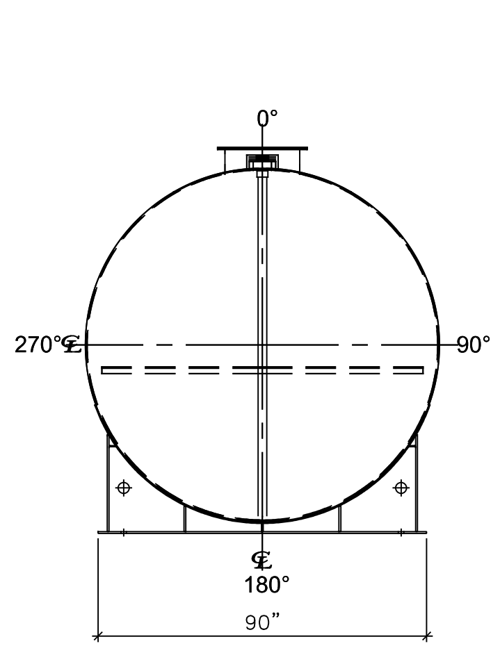
LEFT SIDE
