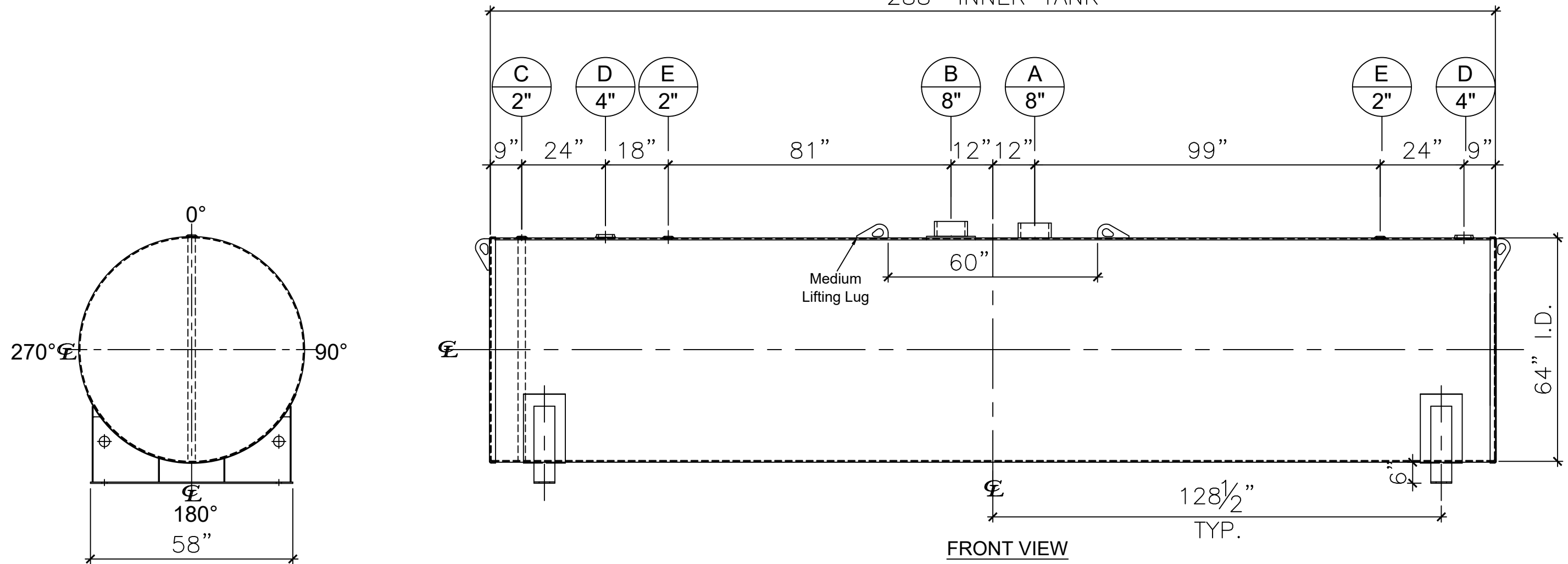
LEFT SIDE
