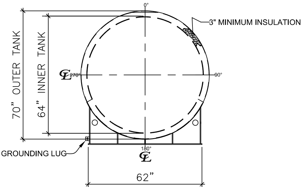
LEFT SIDE
