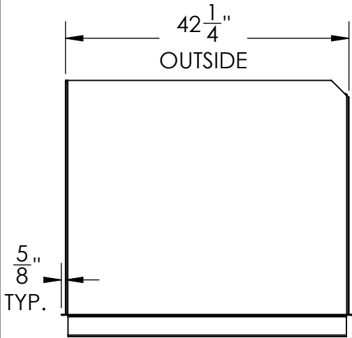
LEFT SIDE
